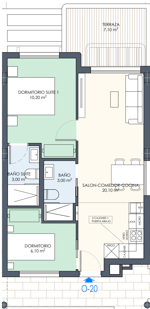
PLANTA PRIMERA
